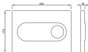
Tehnična risba
