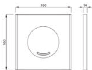
Tehnična risba
